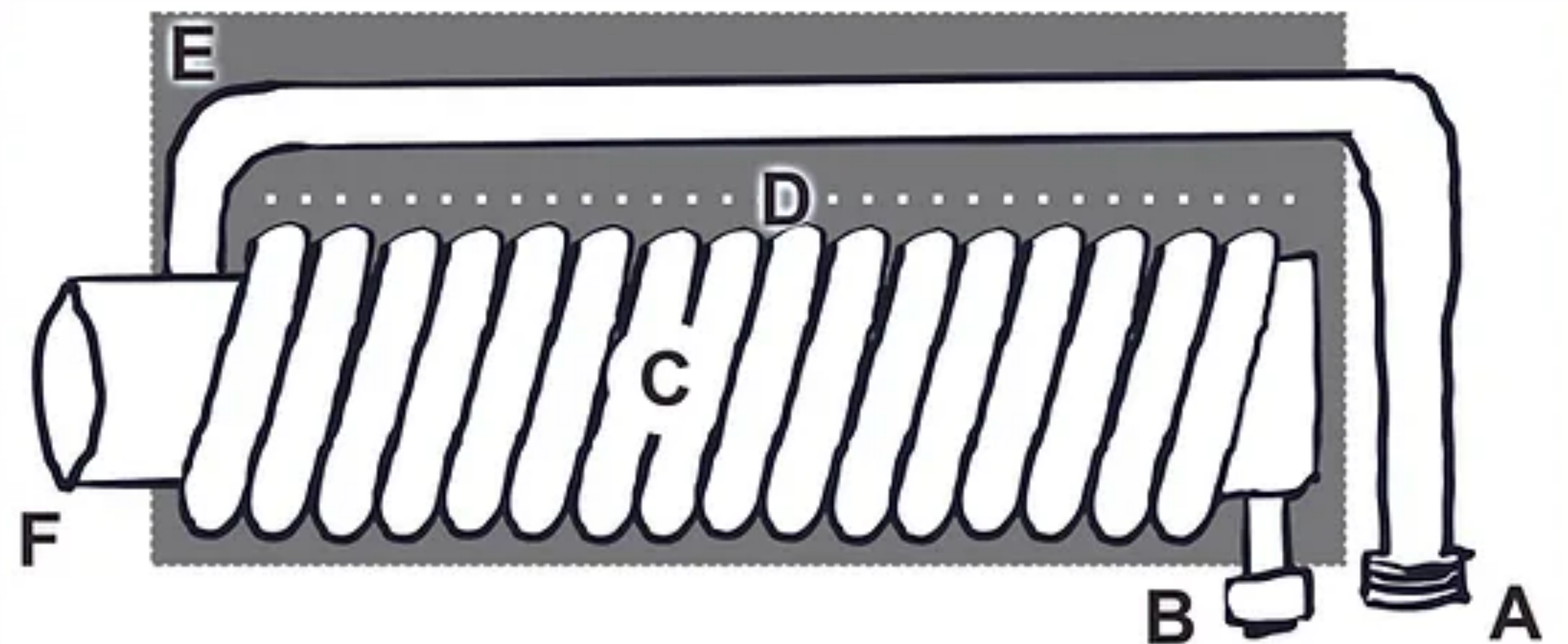
Figura 1. Dorbuster January 5 . A: entrata dell'acqua (tubo di rame da 10-12 mm); B: uscita dell'acqua; C: avvolgimento attorno ad un tubo da 60-80 mm di diametro per creare un flusso di aspirazione del DOR; D: isolamento tra l'entrata dell'acqua ed il flusso in uscita con il DOR assorbito; E: isolamento complessivo dell'apparato; F: estremità del tubo di rame di 6-8 cm di diametro che fa da puntale da applicare sul paziente;
