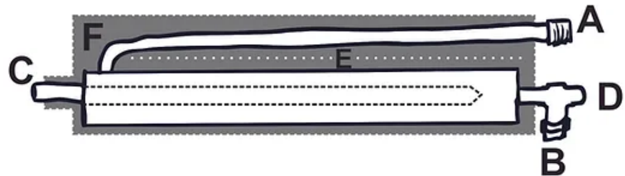
Figura 2. Dorbuster per organopuntura. A: entrata dell'acqua; B: uscita dell'acqua; C: puntale da applicare sul paziente immerso nel flusso acqueo; D: connessione per tubo flessibile di metallo con guaina di plastica per travaso energetico; E: isolamento tra l'entrata dell'acqua ed il flusso in uscita con il DOR assorbito; F: isolamento complessivo dell'apparato.
